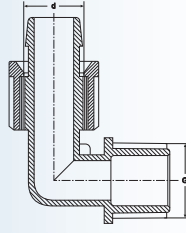
DAMLAMA - ERKEK DİRSEK Dripline - Male Elbow
